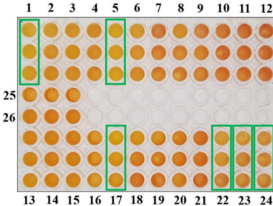
Gambar 1. Fermentasi 24 macam senyawa SFI oleh S. epidermidis . S. epidermidis ATCC 12228 ( 1 \times 10^7 CFU/ml) diinkubasi dengan penambahan 2% 24 senyawa terduga SFI yang berbeda selama 24 jam. Kontrol negatif berupa media RCM tanpa penambahan bakteri dan SFI. Sedangkan kontrol positif berupa media RCM dengan penambahan S. epidermidis ATCC 12228 ( 1 \times 10^7 CFU/ml) dengan dan tanpa penambahan 2% gliserol. Prevalensi fermentasi diindikasikan oleh perubahan warna
