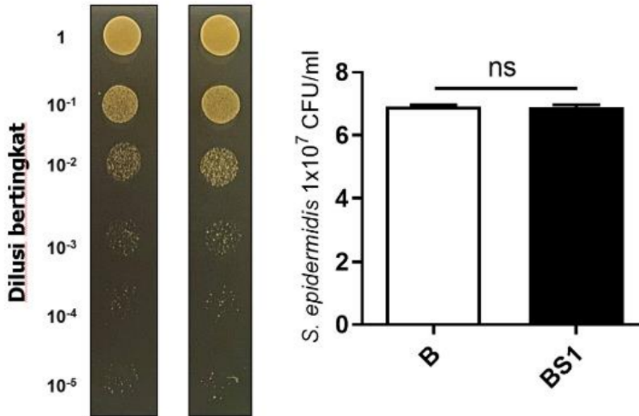
Gambar 7. Tidak adanya efek penghambatan pertumbuhan S. epidermidis ATCC 12228 oleh p-coumaric acid (S1). S. epidermidis ATCC 12228 ( 1 \times 10^7 CFU/ml) diinkubasi dengan dan tanpa 2% p-coumaric acid (selama 12 jam). RCM agar digunakan untuk mendeteksi dan menghitung koloni bakteri setelah didilusi menjadi beberapa tingkat konsentrasi ( 1:10^0 – 1:10^5 ). Rata-rata \pm SE dari hasil diperoleh dari tiga kali percobaan independent. Uji t-test digunakan untuk menentukan signifikansi secara statistik (ns, tidak signifikan).
