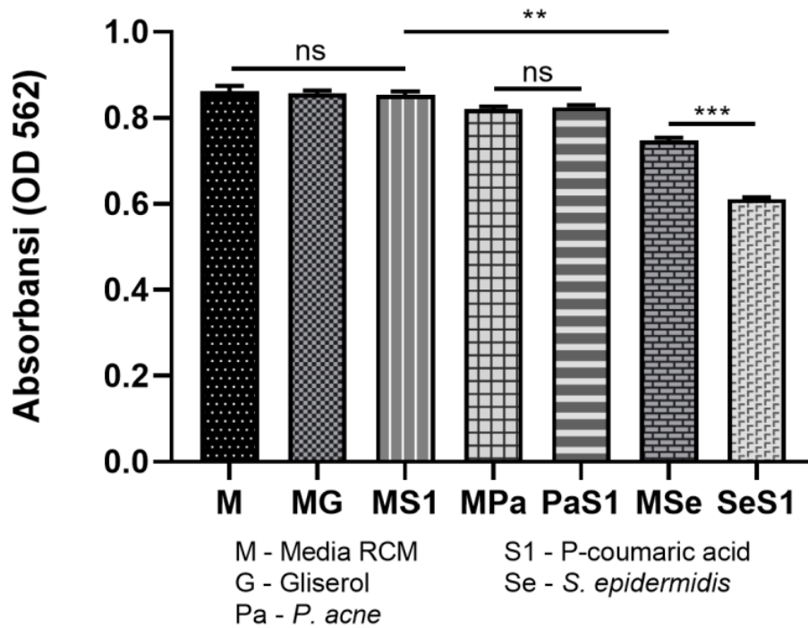
Gambar 4. Pengukuran absorbansi fermentasi 2% p-coumaric acid S. epidermidis dan P. acne . S. epidermidis ATCC 12228 ( 1 \times 10^7 CFU/ml) dan P. acne ( 1 \times 10^7 CFU/ml) diinkubasi dengan dan tanpa penambahan 2% p-coumaric acid. Data merupakan nilai rata-rata \pm SD dari 3 pengulangan uji. *** P < 0,001 ; ** P < 0,05 ; ns tidak signifikan (t-test two tailed).
