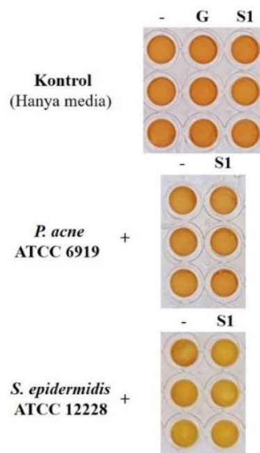
Gambar 3. Fermentasi S. epidermidis ATCC 12228 dan P. acne ATCC 6919 dengan dan tanpa p. coumaric acid (S1). S. epidermidis ATCC 12228 ( 1 \times 10^7 CFU/ml) dan P. acne ATCC 6919 ( 1 \times 10^7 CFU/ml) diinkubasi pada media RCM tanpa dan dengan penambahan 2% p-coumaric acid (S1) selama 24 jam.
