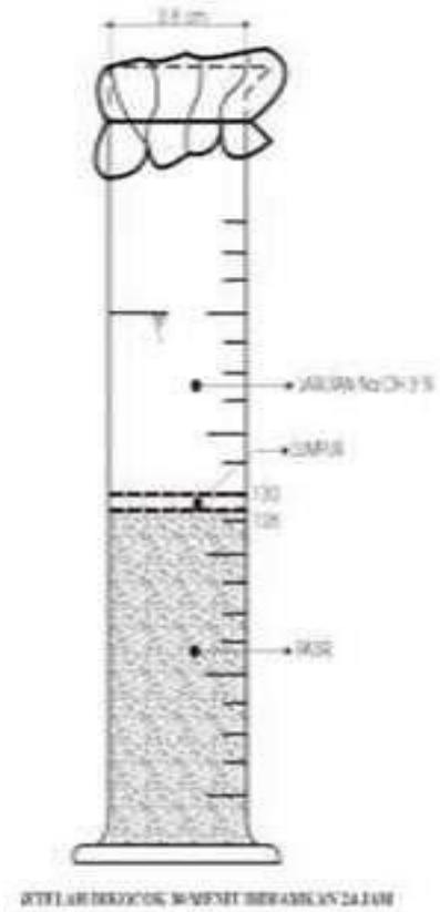
Gambar 1.1 Gelas Ukur dan Percobaan Kadar Lumpur
