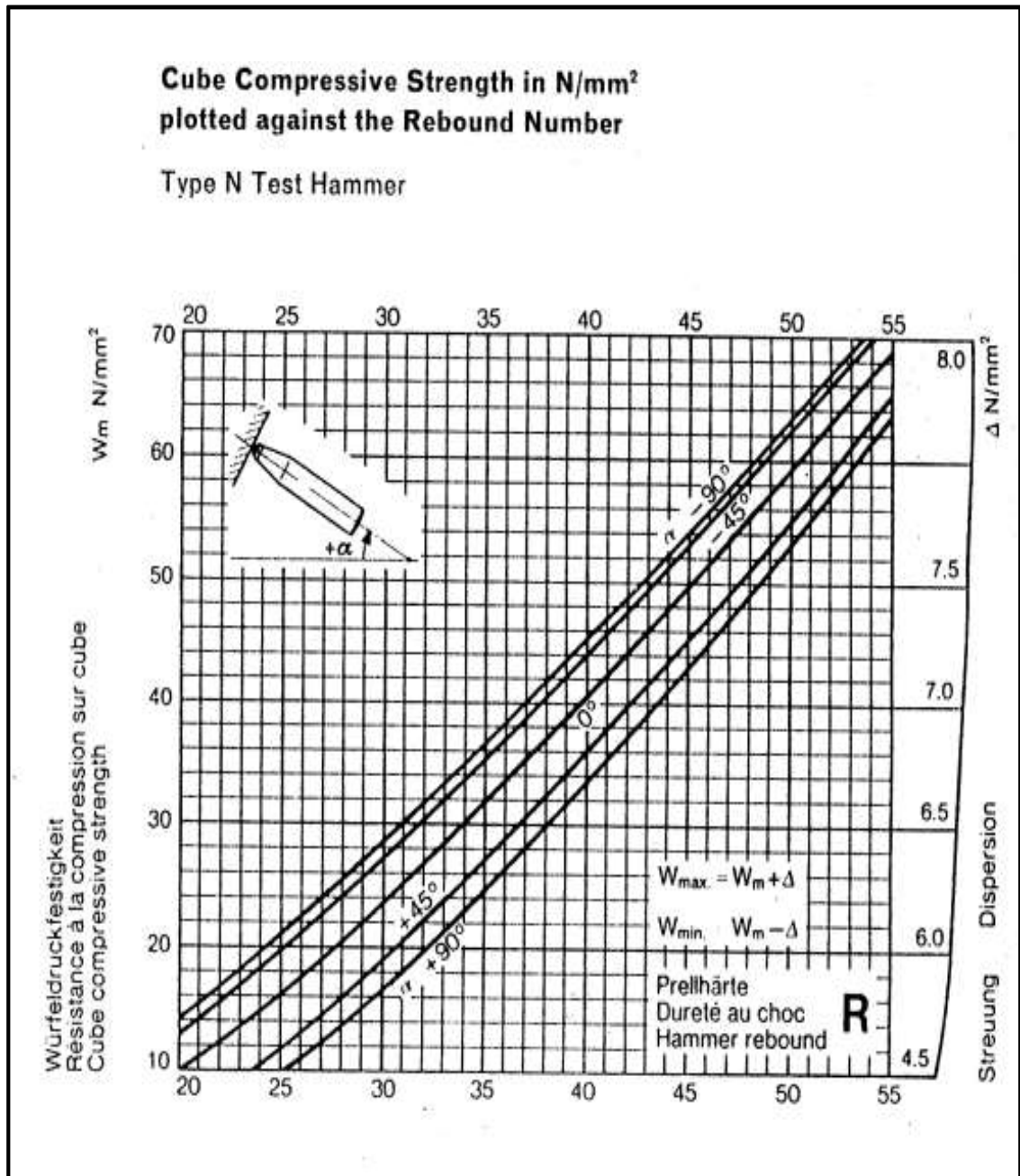
Gambar 3.8. Konversi Rebound Number
