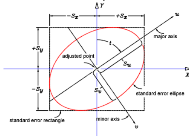
Gambar 2.2. Ellips Kesalahan
