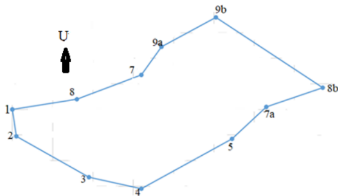
Gambar 4.1. Bentuk Jaring Poligon
