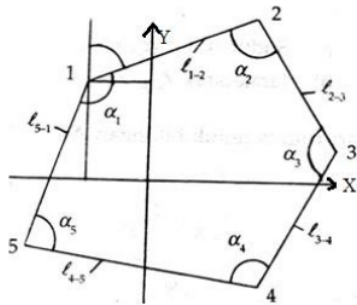
Gambar 2.1. Poligon Tertutup Segilima
