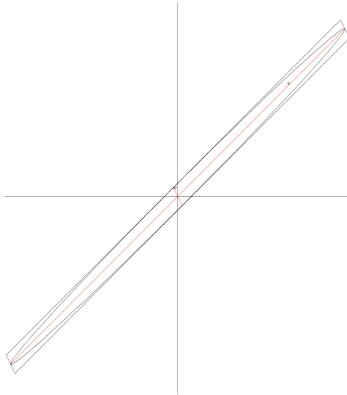
Gambar 5. Ellips Kesalahan Poligon Stasiun 5
