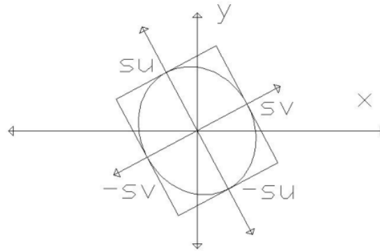
Gambar 2.4. Bentuk Ellips Kesalahan Pemotongan Kebelakang
