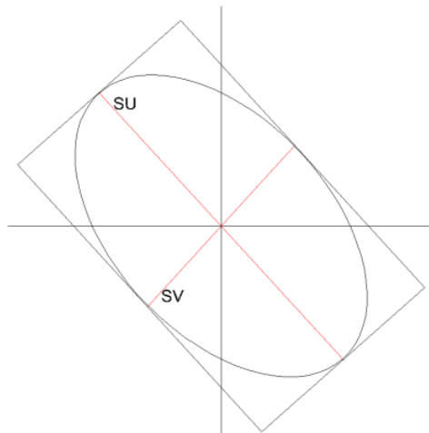
Gambar 2. Ellips Kesalahan Poligon Stasiun 2
