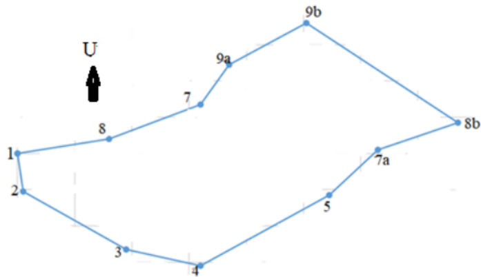
Gambar 3.1. Bentuk Jaring Poligon
