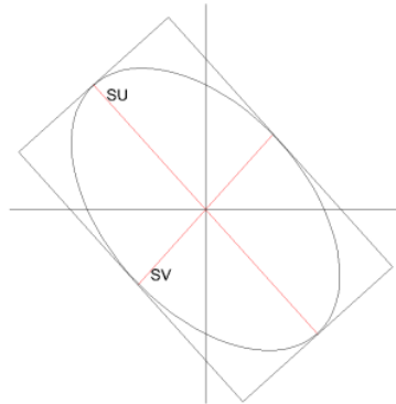
Gambar 4.2. Ellips Kesalahan Poligon Stasiun 2
