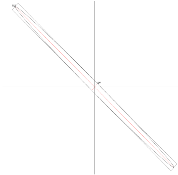
Gambar 7. Ellips Kesalahan Poligon Stasiun 8b
