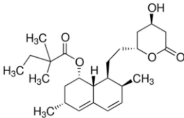
Gambar 9. Struktur simvastatin
