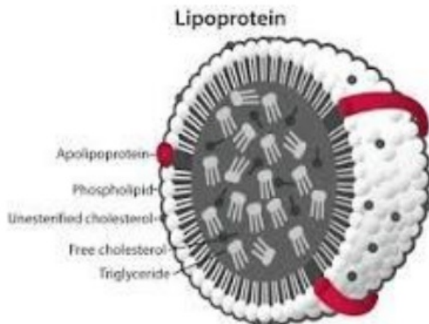
Gambar 4. Struktur lipoprotein
