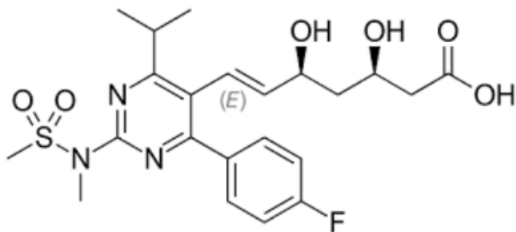
Gambar 12. Struktur rosuvastatin
