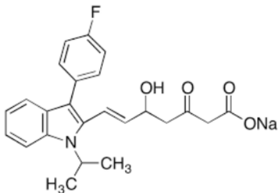
Gambar 11. Struktur fluvastatin
