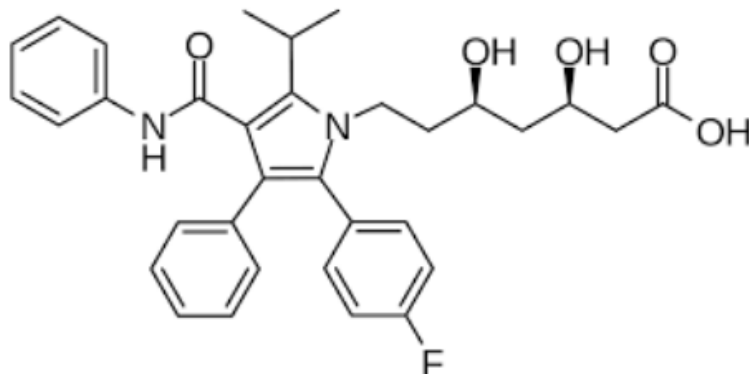
Gambar 15. Struktur atorvastatin
