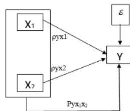
Gambar 1. Diagram Jalur Antar Variabel
