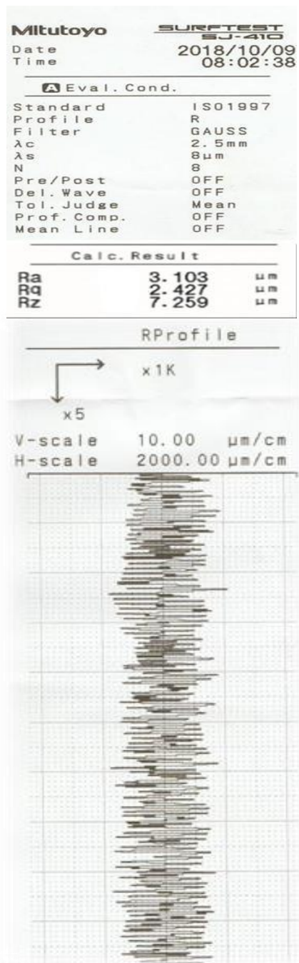
Gambar L.9. Hasil pengukuran kekasaran pada sample 9
