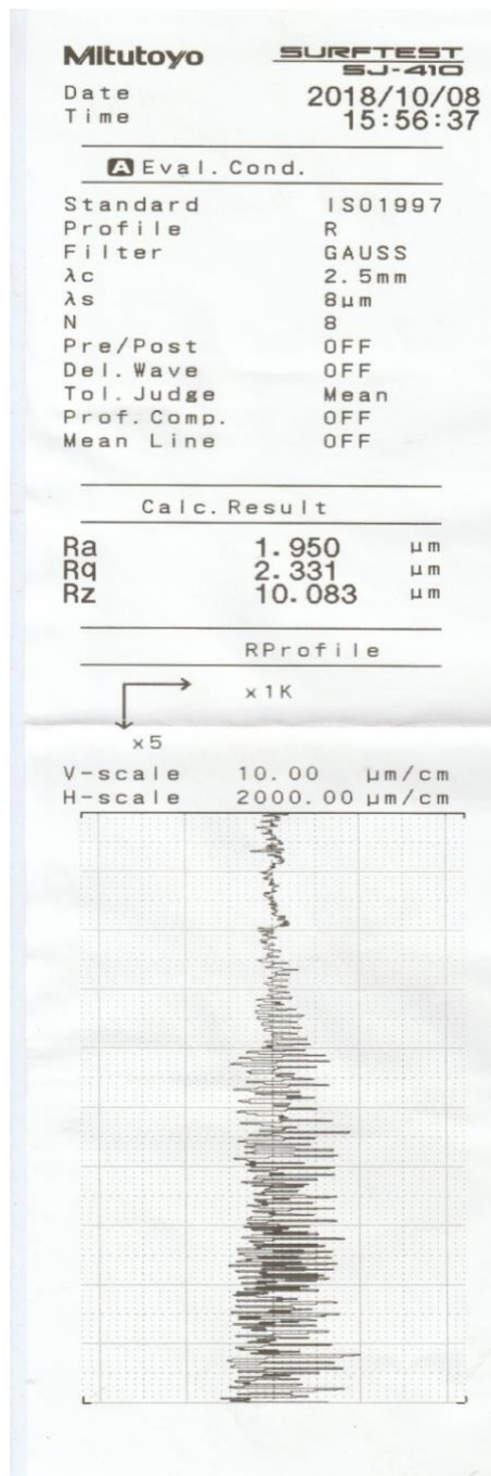
Gambar L.7. Hasil pengukuran kekasaran pada sample 7
