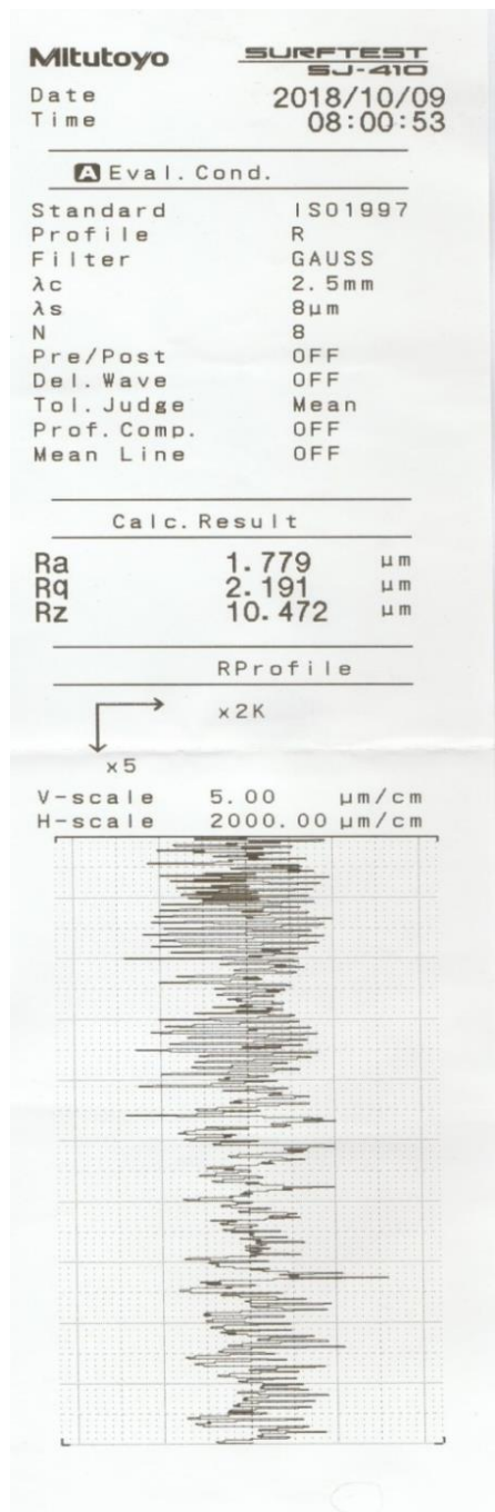
Gambar L.3. Hasil pengukuran kekasaran pada sample 3
