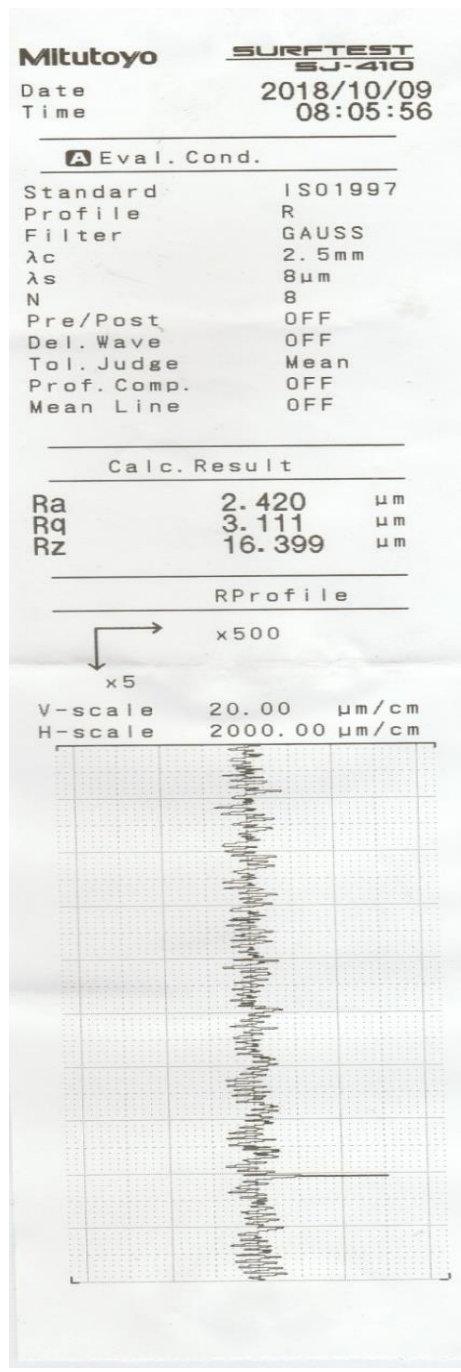
Gambar L.6. Hasil pengukuran kekasaran pada sample 6
