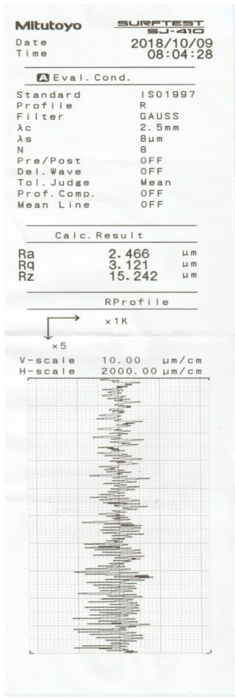
Gambar L.4. Hasil pengukuran kekasaran pada sample 4
