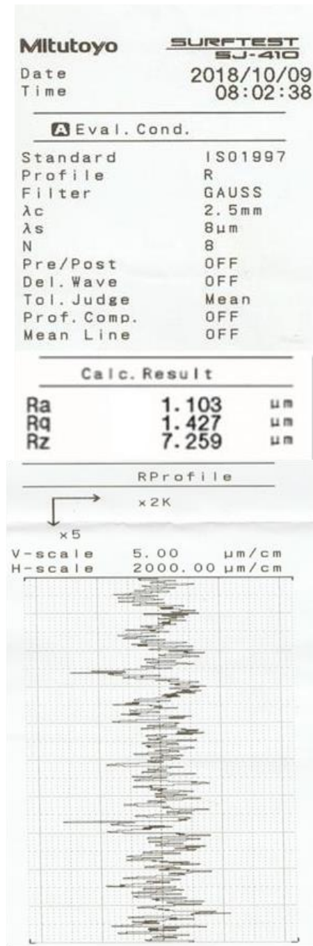
Gambar L.1. Hasil pengukuran kekasaran pada sample 1
