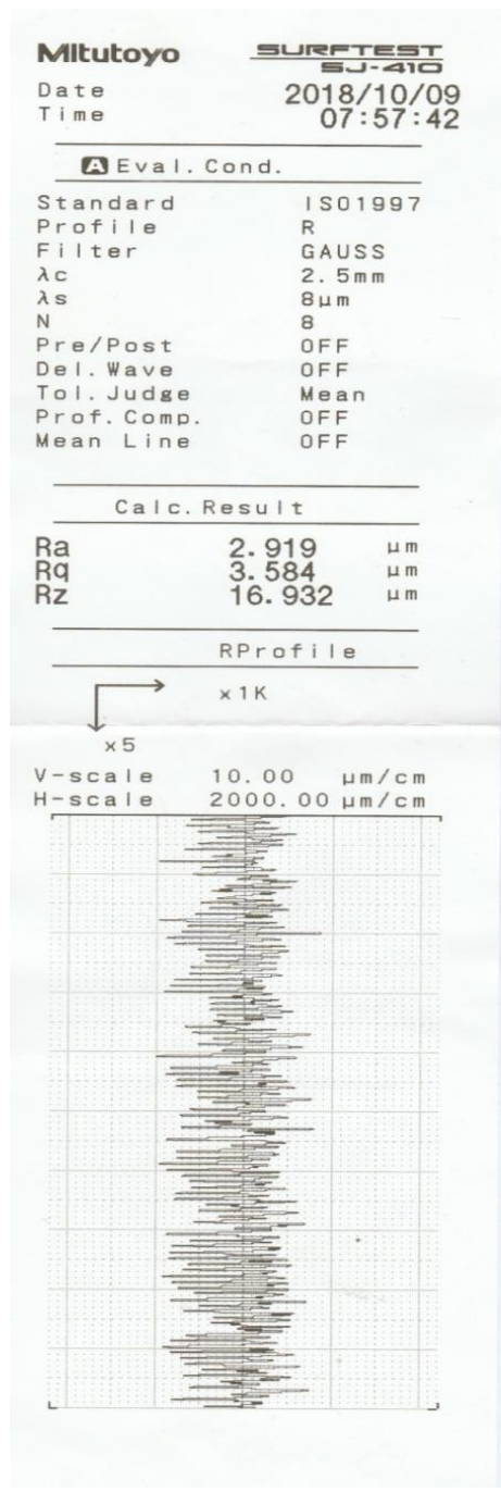
Gambar L.8. Hasil pengukuran kekasaran pada sample 8
