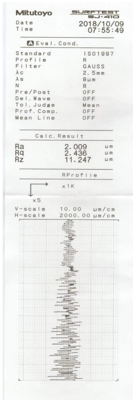
Gambar L.2. Hasil pengukuran kekasaran pada sample 2
