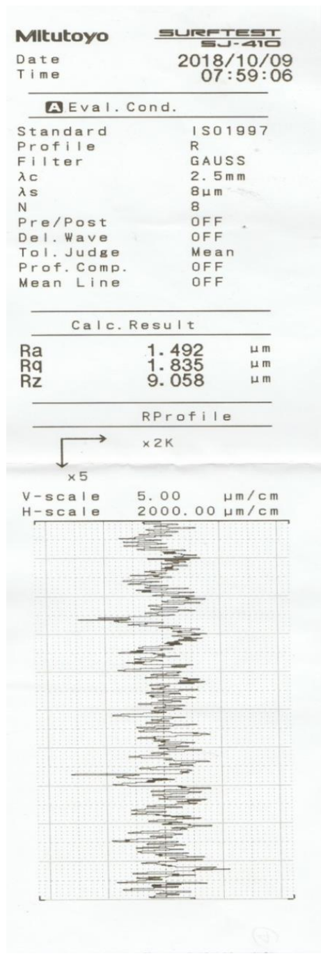
Gambar L.5. Hasil pengukuran kekasaran pada sample 5
