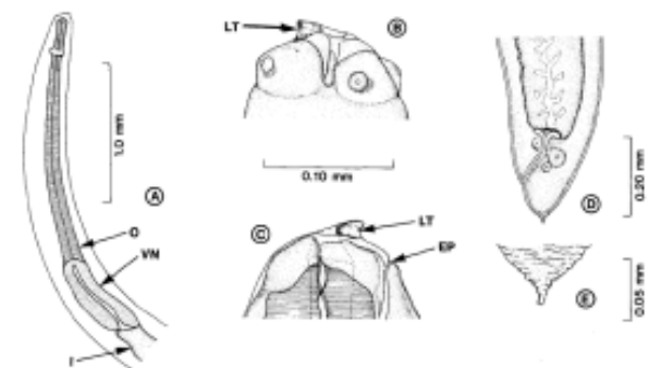
Gambar 3. Skema larva III Anisakis simplex . A aspek anterior, B aspek lateral, C aspek sagittal, D aspek postero-lateral, E perbesaran ekstremitas posterior, tampak mucron. LT=lateral tooth/gigi lateral, EP=excretory pore/porus ekskretorius, IC= intestinal caecum/caecum intestinal, O=oesophagus, VN=ventriculus. 24 dengan modifikasi
