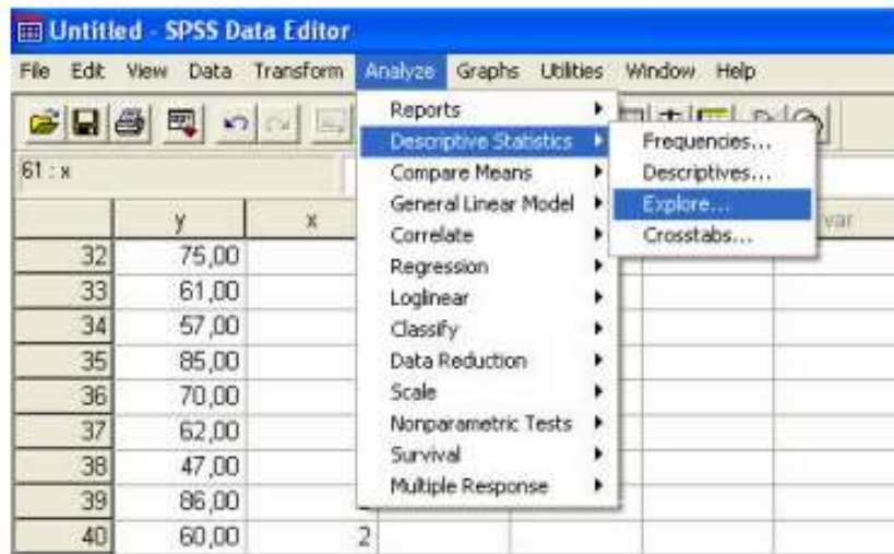
Gambar 4 Tampilan Perintah Uji Normalitas
