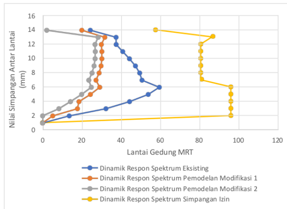
Gambar 9. Simpanan Antar Lantai Statik Ekuivalen Pemodelan 2 Shear wall arah X
