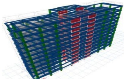
Gambar 4. Pemodelan 3D Shear wall Modifikasi 1
