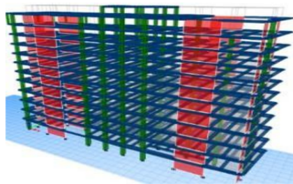
Gambar 6. Pemodelan 3D Shear wall Modifikasi 2
