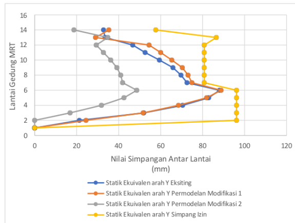
Gambar 8. Simpanan Antar Lantai Dinamik Pemodelan 1 Shear wall arah Y
