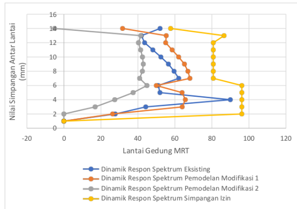
Gambar 10. Simpangan Antar Lantai Dinamik Pemodelan 2 Shear wall arah Y
