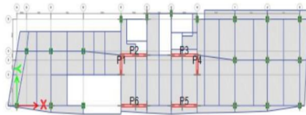
Gambar 3. Denah Shear wall Modifikasi 1
