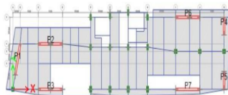
Gambar 5. Denah Shear wall Modifikasi 2
