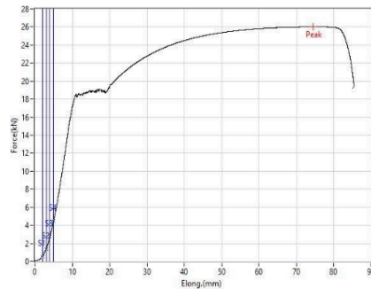
Gambar 7. Uji Kuat Tarik Baja
