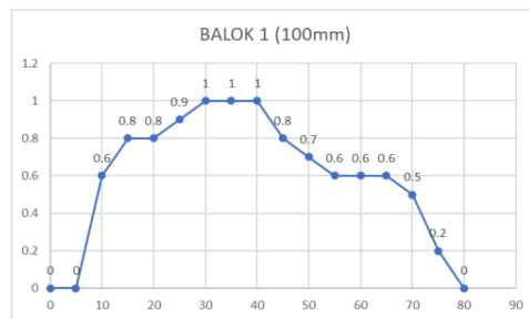
Gambar 9. Lendutan Balok B1
