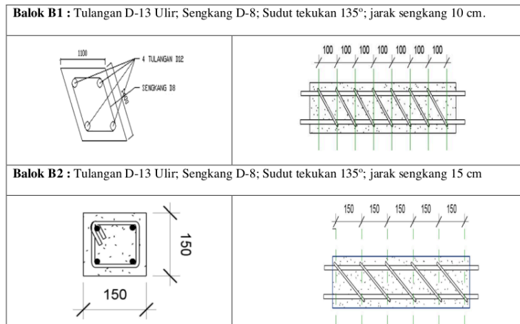
Gambar 3. Detail Desain Tulangan Balok B-1 dan Balok B-2
