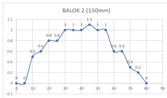
Gambar 10. Lendutan Pada Balok B2
