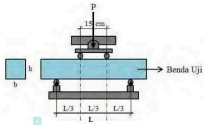
Gambar 1. Pengujian Balok Beton Bertulang dengan 1 Titik
