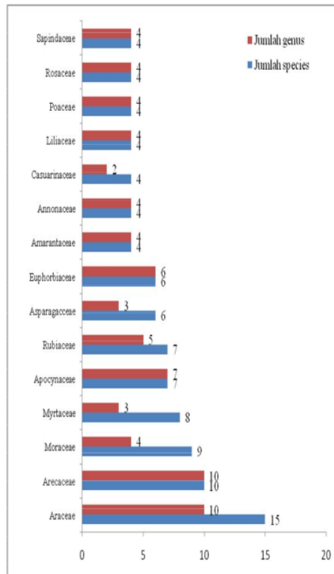
Gambar 1. Komposisi tumbuhan di nursery Kranggan dengan famili yang memiliki jumlah spesies terbanyak.
