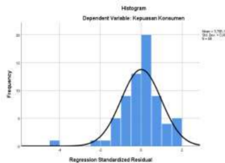
GAMBAR 4.1 UJI NORMALITAS HISTOGRAM
