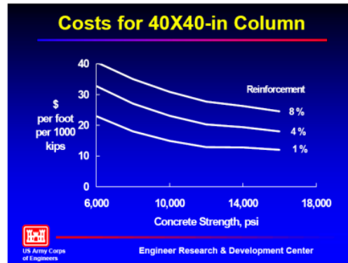
Gambar 7: Hubungan Biaya dan Kuat tekan beton mutu Tinggi pada kolom (Sumber : V.M Malhotra, 2002)
