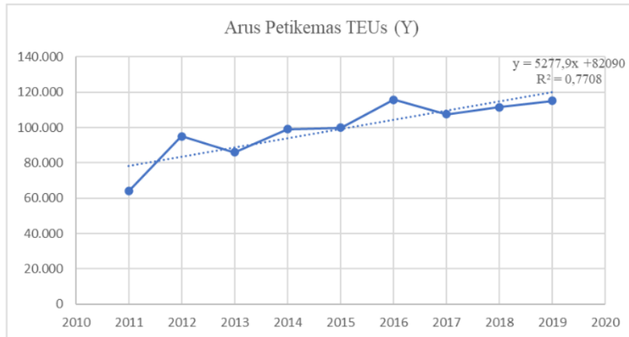
Gambar 2 Grafik arus peti kemas Pelabuhan Tenau Kupang tahun 2011 s/d 2019
