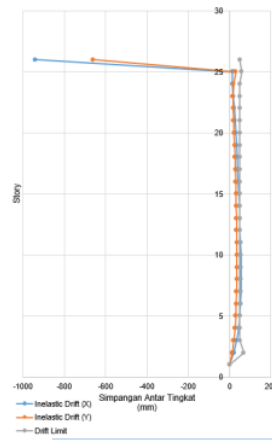
Gambar 8. Simpangan Antar Tingkat Akibat Beban Gempa California
