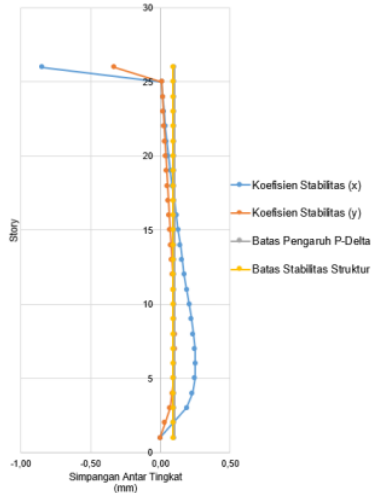
Gambar 10. Pengaruh P-Delta Akibat Beban Gempa Respon Spektrum
