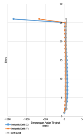
Gambar 9. Simpangan Antar Tingkat Akibat Beban Gempa San Francisco
