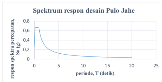
Gambar 2. Respon Spektar Pada Tanah Lunak (SE)
