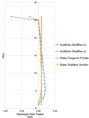
Gambar 11. Pengaruh P-Delta Akibat Beban Gempa Kobe
