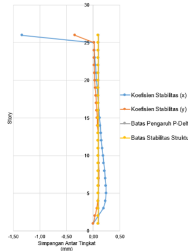
Gambar 13. Pengaruh P-Delta Akibat Beban Gempa San Francisco
