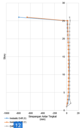
Gambar 7. Simpangan Antar Tingkat Akibat Beban Gempa Kobe
