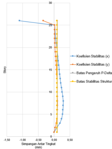
Gambar 12. Pengaruh P-Delta Akibat Beban Gempa California
