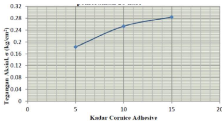
Gambar 5. Hasil pengujian Tegangan aksial vs kadar CA pada pemeraman 28 hari (Hebron et al., 2022)
