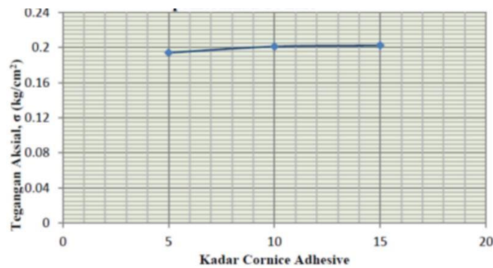
Gambar 4. Hasil pengujian Tegangan aksial vs kadar CA pada pemeraman 14 hari (Hebron et al., 2022)
