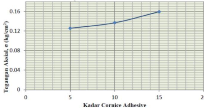
Gambar 3. Hasil Pengujian Tegangan aksial vs Kadar Cornice Adhesive pada pemeraman 7 hari (Hebron et al., 2022)
