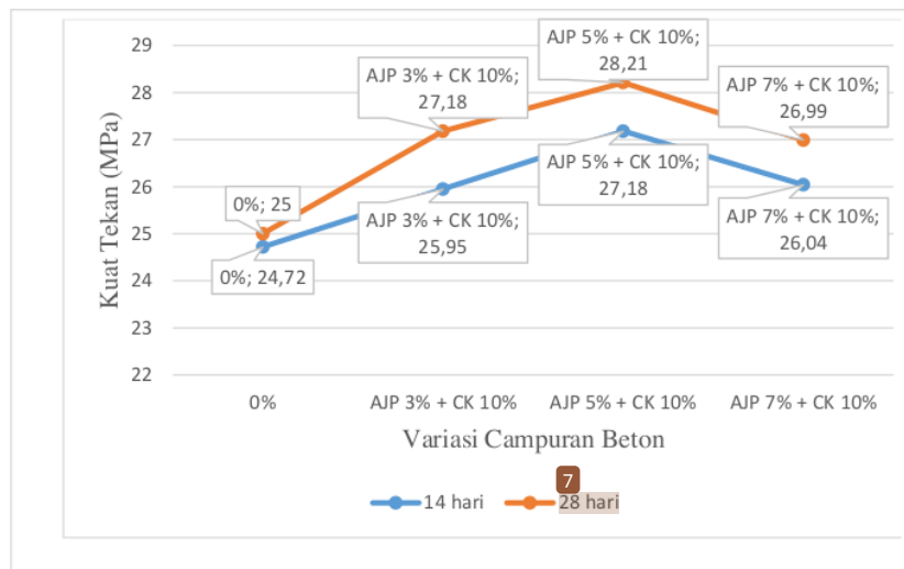
Gambar 1. Hasil Uji Tekan Beton
