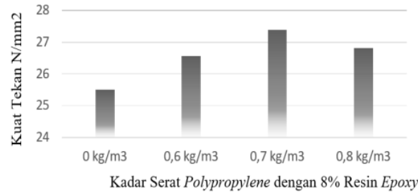
Gambar 5. Penambahan Serat Polypropylene dan Epoxy Resin Terhadap Kuat Tekan Beton umur 14 hari
