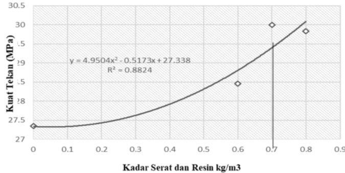
Gambar 6. Peningkatan Kuat Tekan Beton Umur 28 hari
