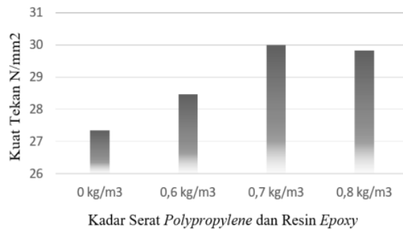
Gambar 6. Penambahan Serat Polypropylene dan Epoxy Resin Terhadap Kuat Tekan Beton umur 28 hari
