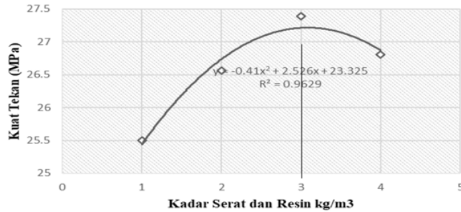
Gambar 5. Peningkatan Kuat Tekan Beton Umur 14 hari
