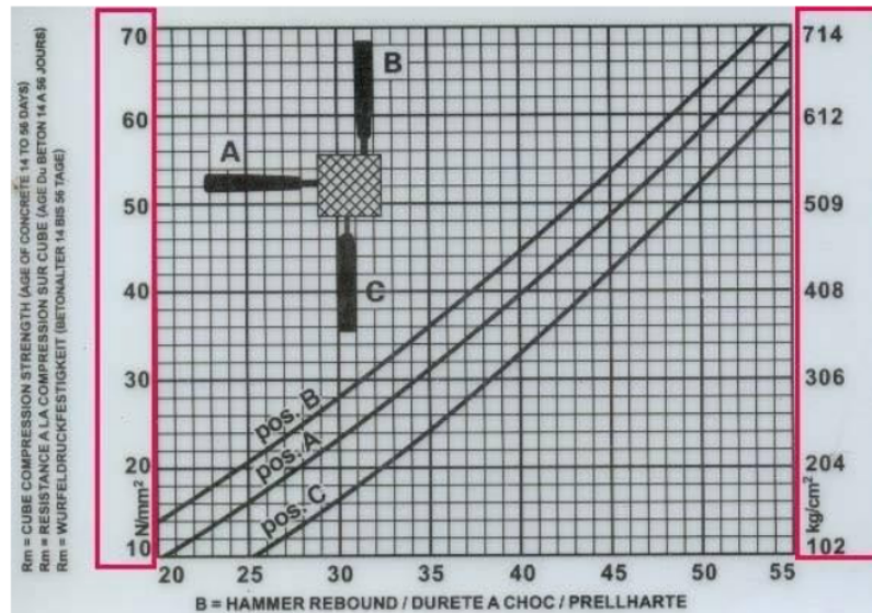
Gambar 4. Grafik Hammer Test
