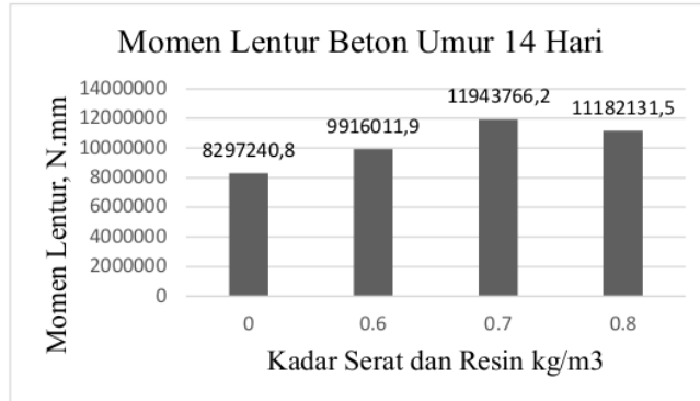
Gambar 7. Peningkatan Peningkatan Momen Lentur Beton umur 14 hari
