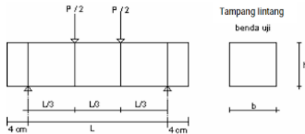
Gambar 3. Uji Momen Lentur (Sumber: ACI 440.1R-15)
