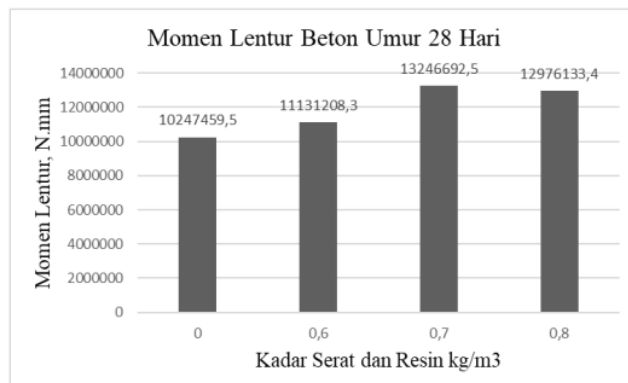
Gambar 8. Peningkatan Peningkatan Momen Lentur Beton umur 28 hari
