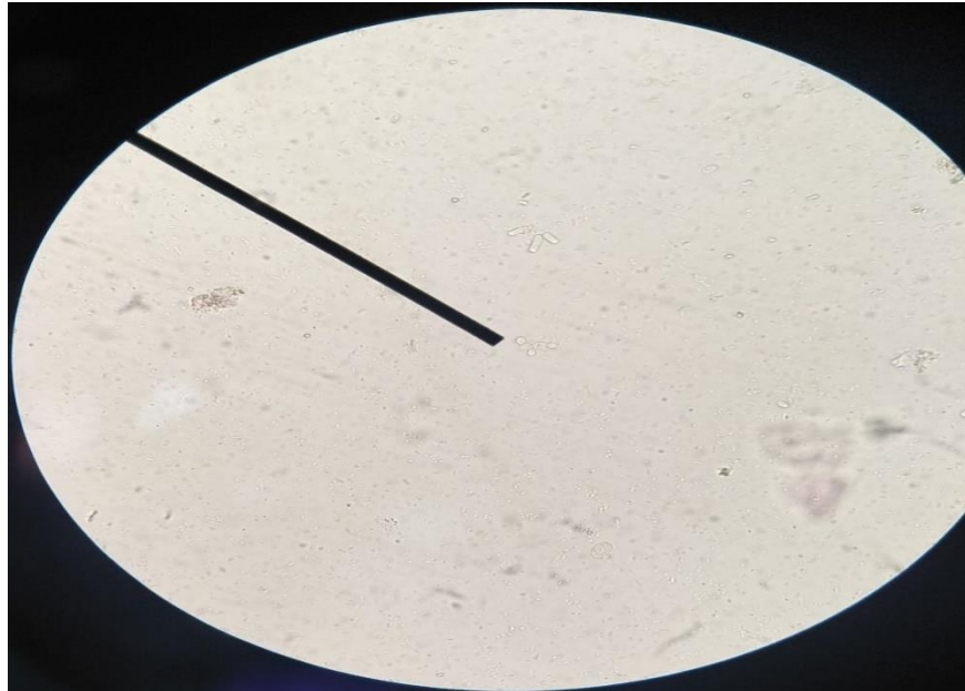
Gambar VI.3. spora jamur
