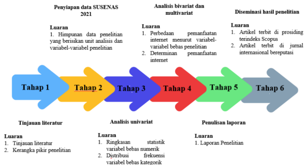
Gambar 1. Tahapan Penelitian
